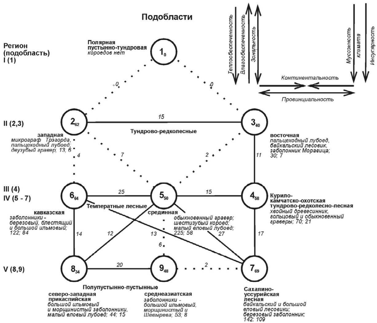
Рис. 2. Пространственно-типологическая структура фауны короедов Северной Евразии на уровне подобласти. Внутри значков приведены номера таксонов соответствующей классификации, индексом — внутригрупповое сходство. Сплошные линии между значками означают существенное сверхпороговое сходство, пунктирные линии — запороговое. Около этих линий обозначены значения межгруппового сходства. Около значков, кроме наименования подобластей, приведены названия трёх лидирующих видов короедов, общее число отмеченных видов и средняя суммарная встречаемость. Стрелки около перечня основных структурообразующих факторов среды указывают направление увеличения их влияния и фаунистические тренды
